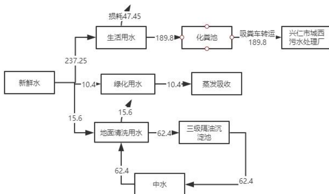
2-2 项目水平衡图 (t/a)
